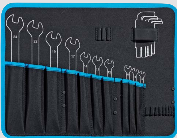
Individueller Konturendruck Ihres Werkzeugsortiments individual lineprinting of your tool assortment
